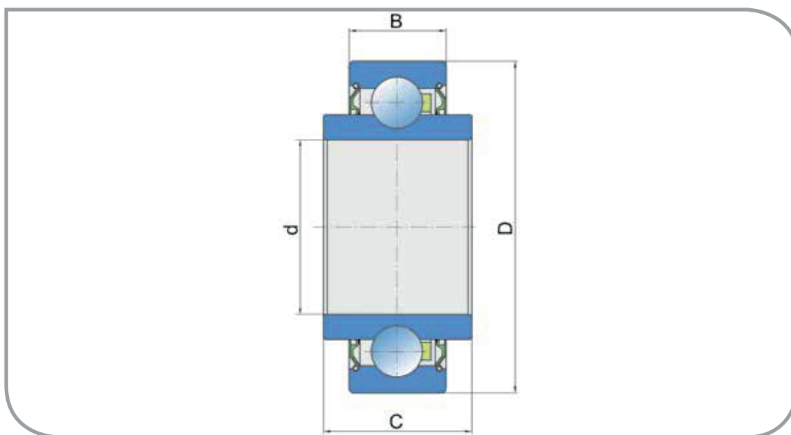
Abmessungen/Dimensions (mm)
