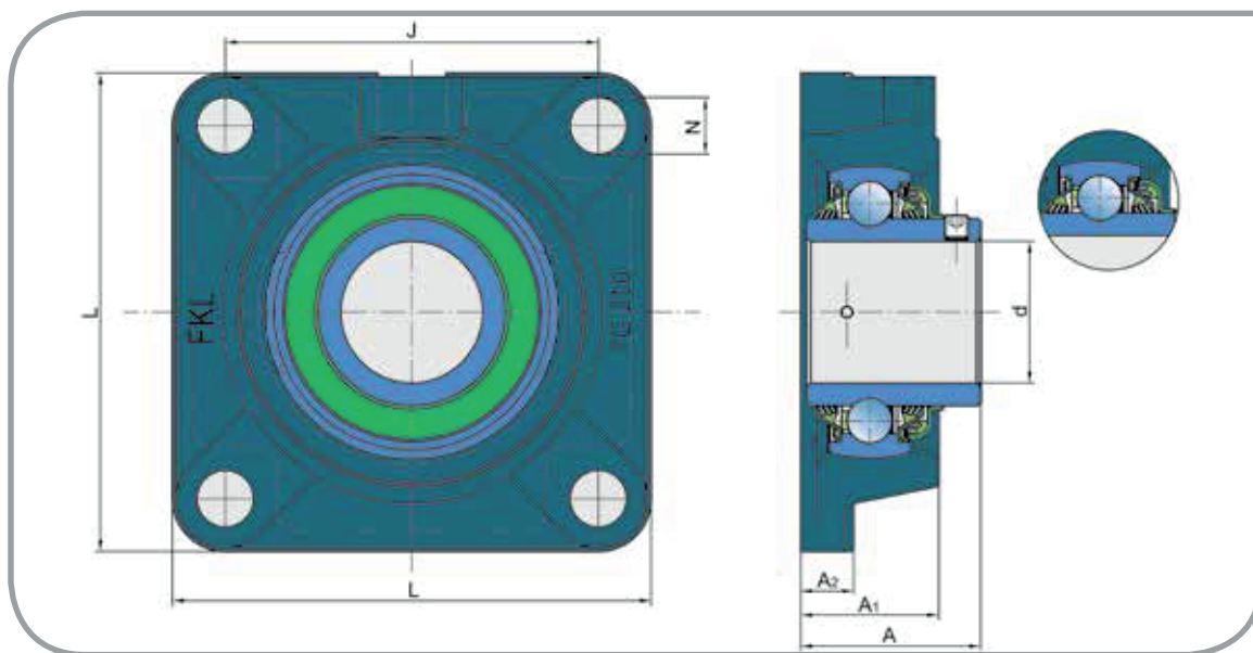
Abmessungen/Dimensions (mm)
