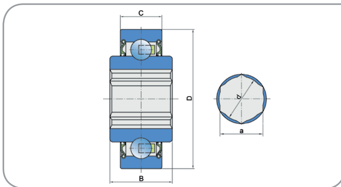
Abmessungen/Dimensions (mm)
