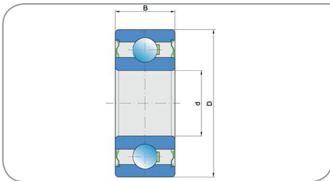
Abmessungen/Dimensions (mm)
