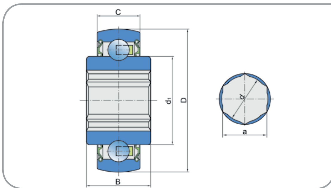
Abmessungen/Dimensions (mm)
