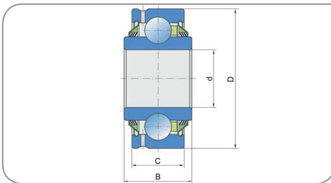
Abmessungen/Dimensions (mm)
