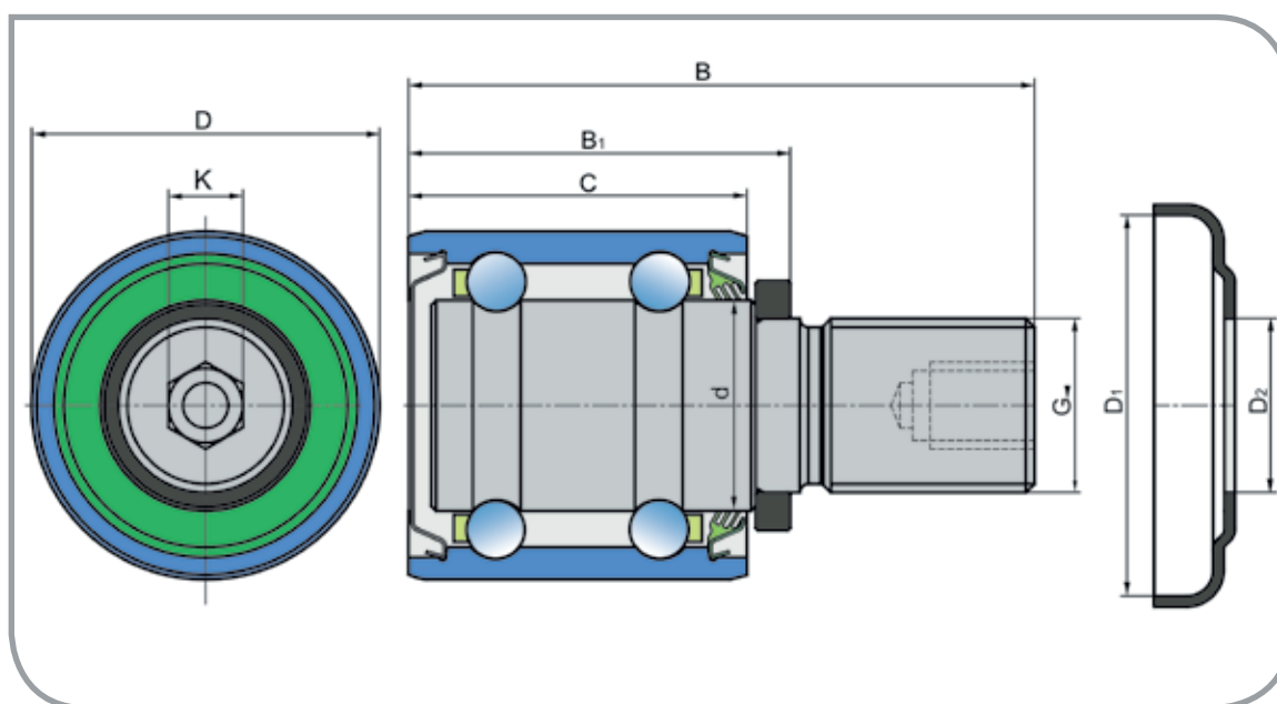
Abmessungen/Dimensions (mm)
