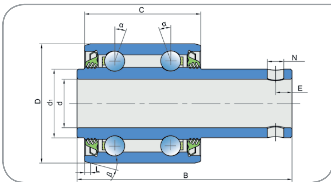
Abmessungen/Dimensions (mm)
